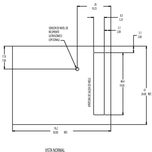
Vista superior - Todos
