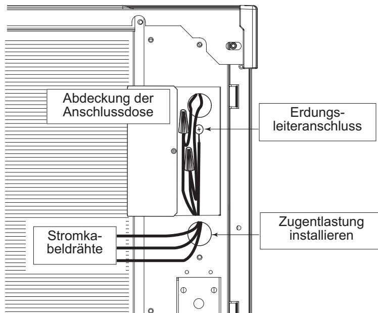
Elektrische Anschlüsse, Geräterückseite
