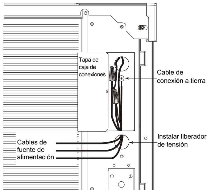
Conexiones eléctricas, parte posterior de la unidad
