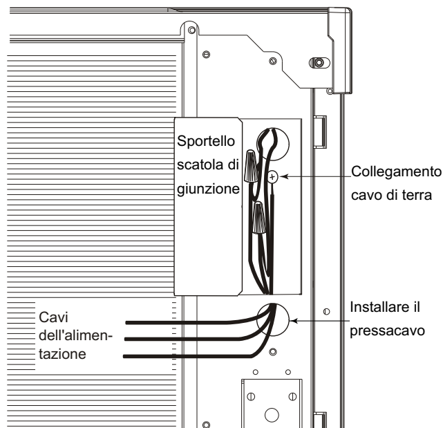
Collegamenti elettrici, retro dell'unità
