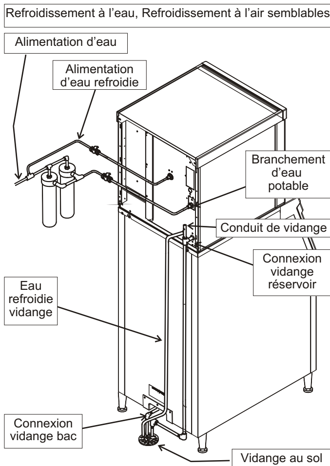
Raccords de plomberie
