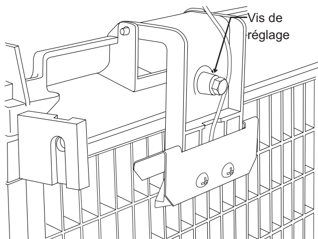
Mécanisme de réglage de l'épaisseur de jonction
