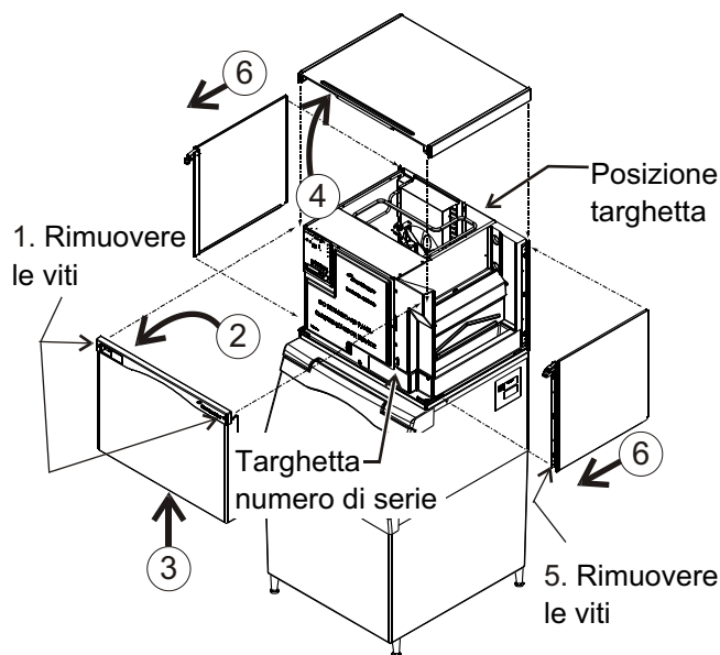
Posizione targhetta delle caratteristiche e rimozione pannelli
