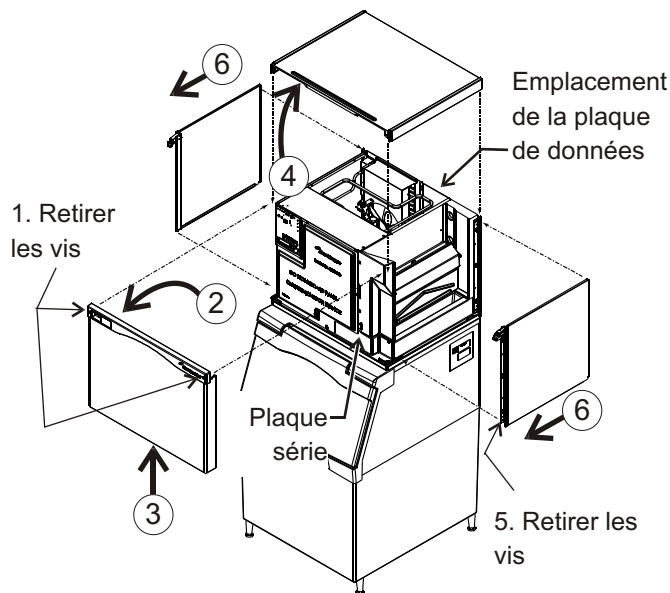
Emplacement de la plaque d'information et retrait du panneau
