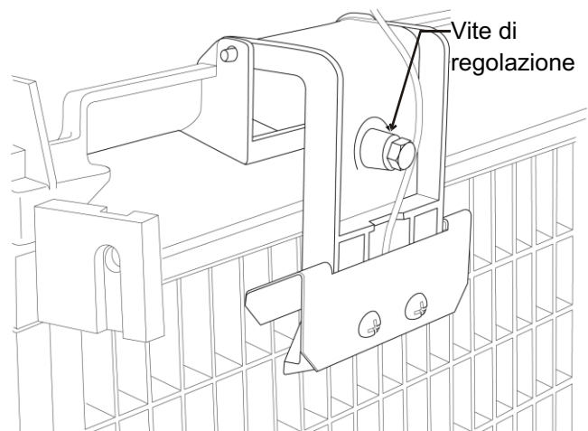
Meccanismo regolazione spessore ghiaccio
