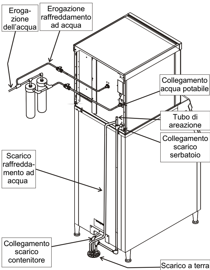
Collegamenti idraulici
