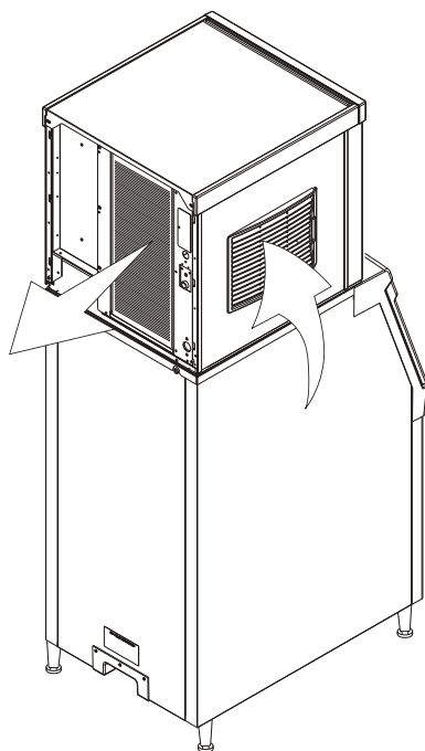
Flusso dell'aria
