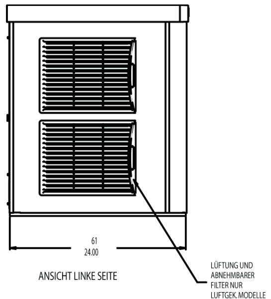
C0830, C1030 Seitenansicht luftgekühlter Modelle
