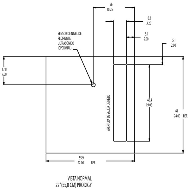
Vista superior
