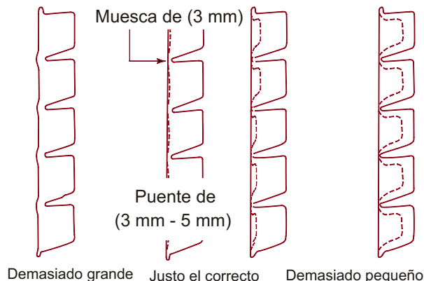
Medición del grosor del puente de hielo
