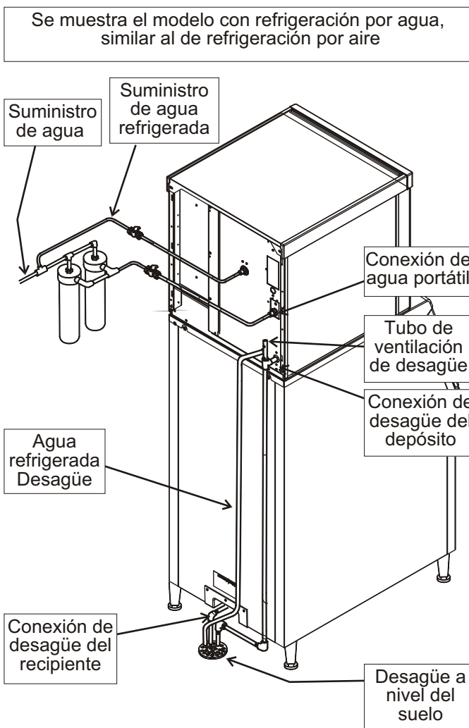
Conexiones de fontanería
