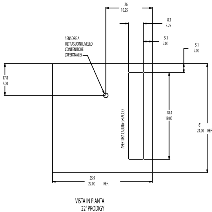
Vista superiore
