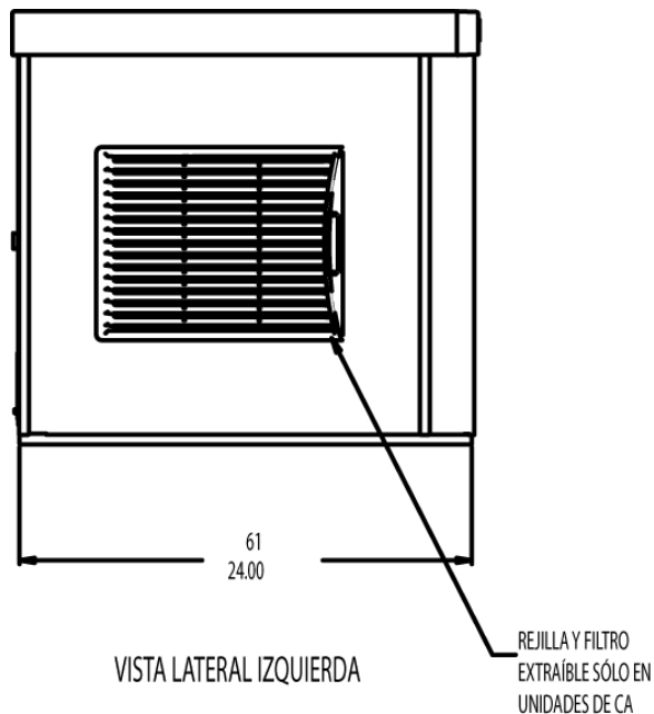
Vista lateral del modelo con refrigeración por aire C0330, C0530, C0630
