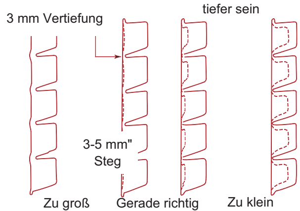
Messung der Eisstegdicke
