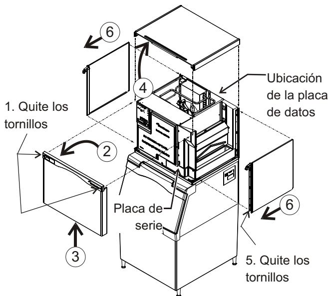
Ubicación de placa de datos y desmontaje del panel
