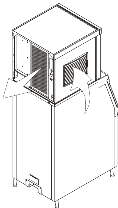
Circulación del aire
