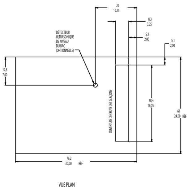
VUE PLAN
