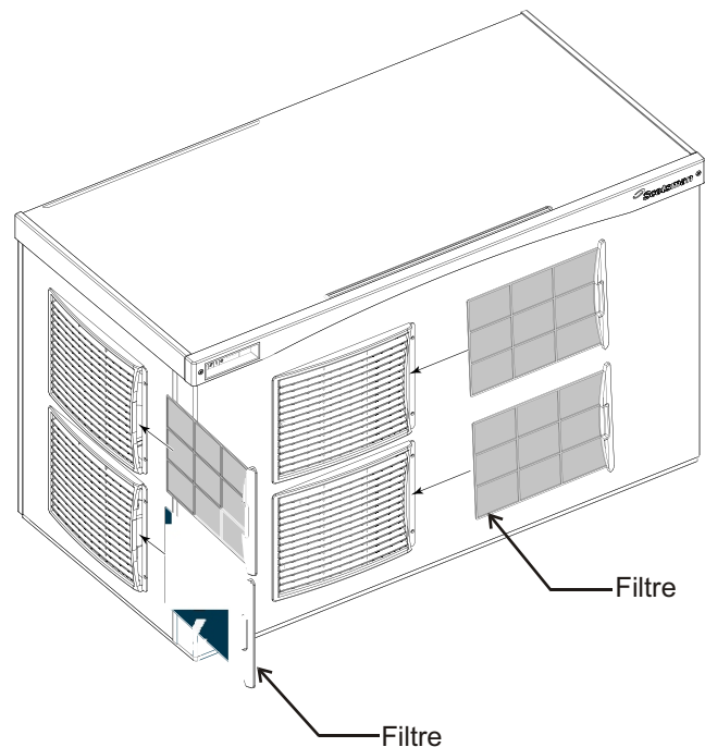
Retrait du filtre à air
