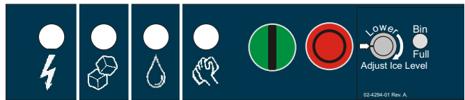
Área de control Vari-Smart
