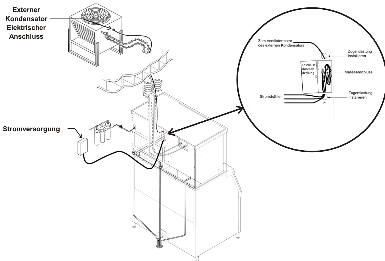
Elektrische Anschlüsse
