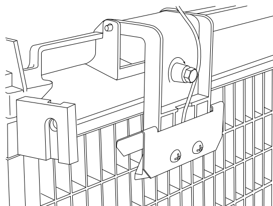
Décteur de l'épaisseur des glaçons
