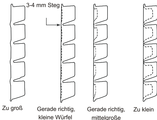
Messung der Eisstegdicke
