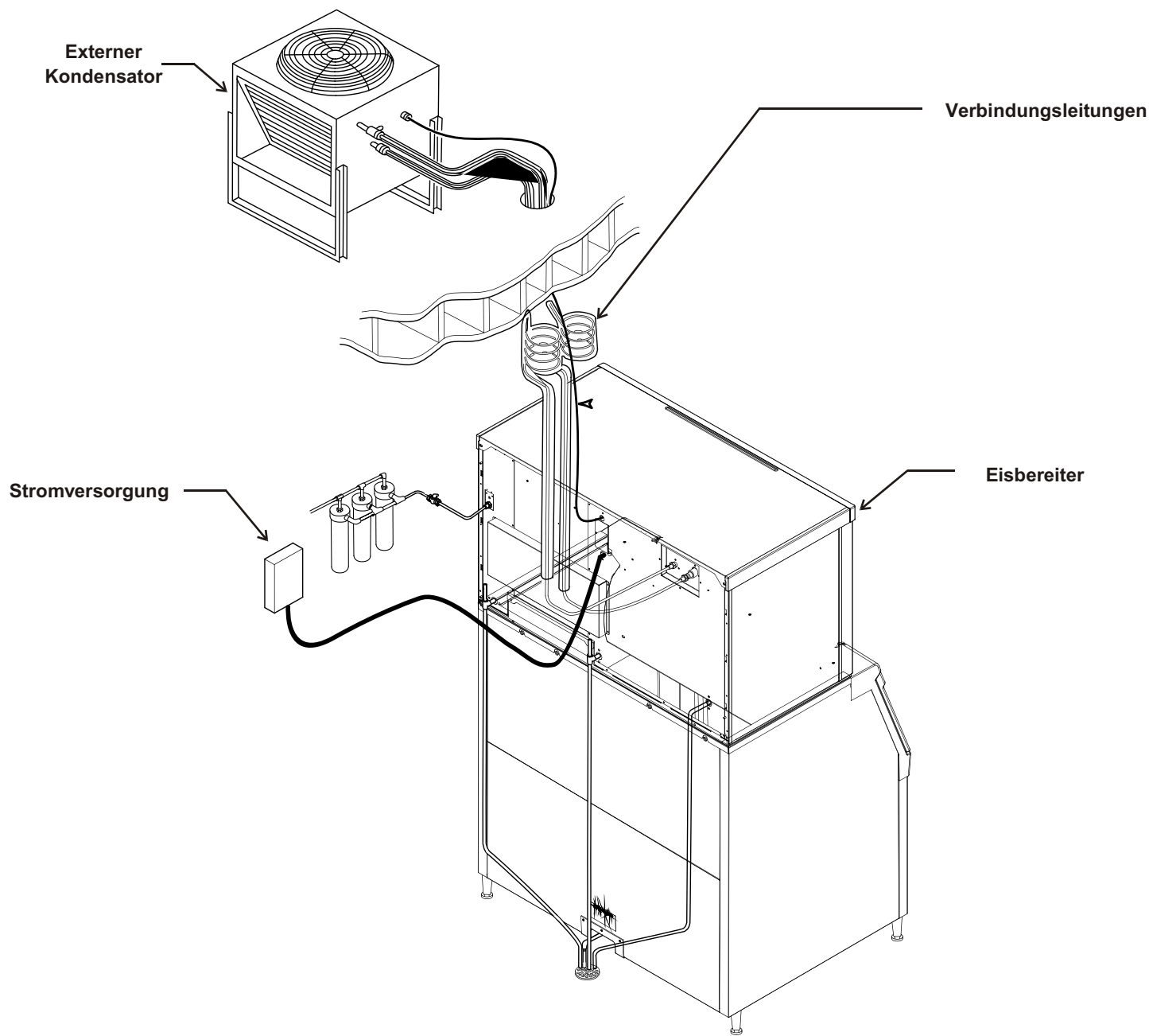
Externer Kondensator, Abbildung eines typischen Systems
