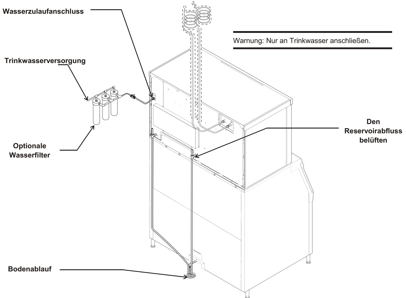
Wasserversorgungs- und Abflussanschlüsse
