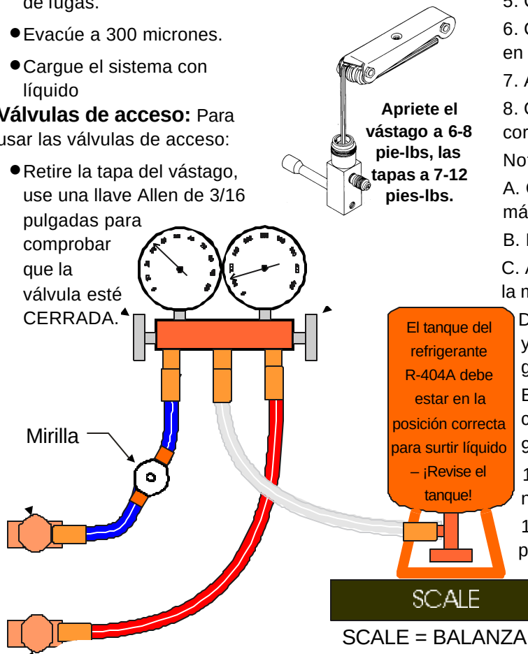
Plano de conexión de mangueras para cargar líquido
